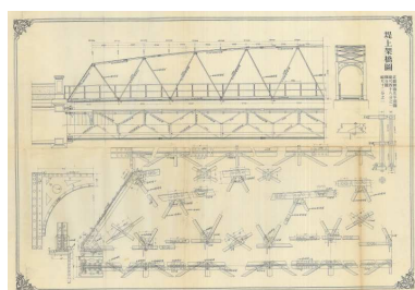
堤上架橋図 (藤倉水源地) (資料提供：秋田市上下水道局)
