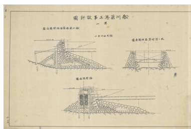
船川築港工事設計図その一 (資料提供：船川港湾事務所)
