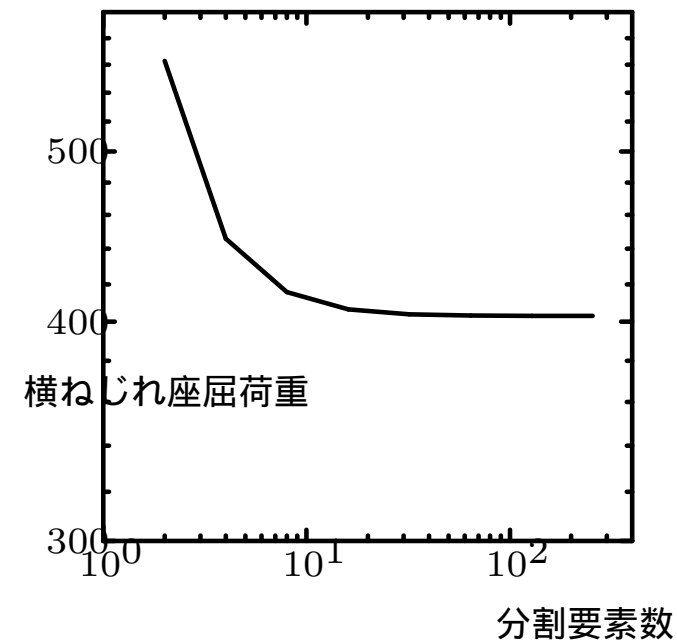
分割要素数と横ねじれ座屈荷重の関係
