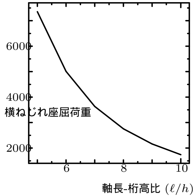
細長比と横ねじれ座屈荷重の関係
